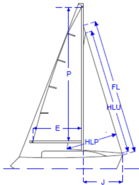
SLOOP
